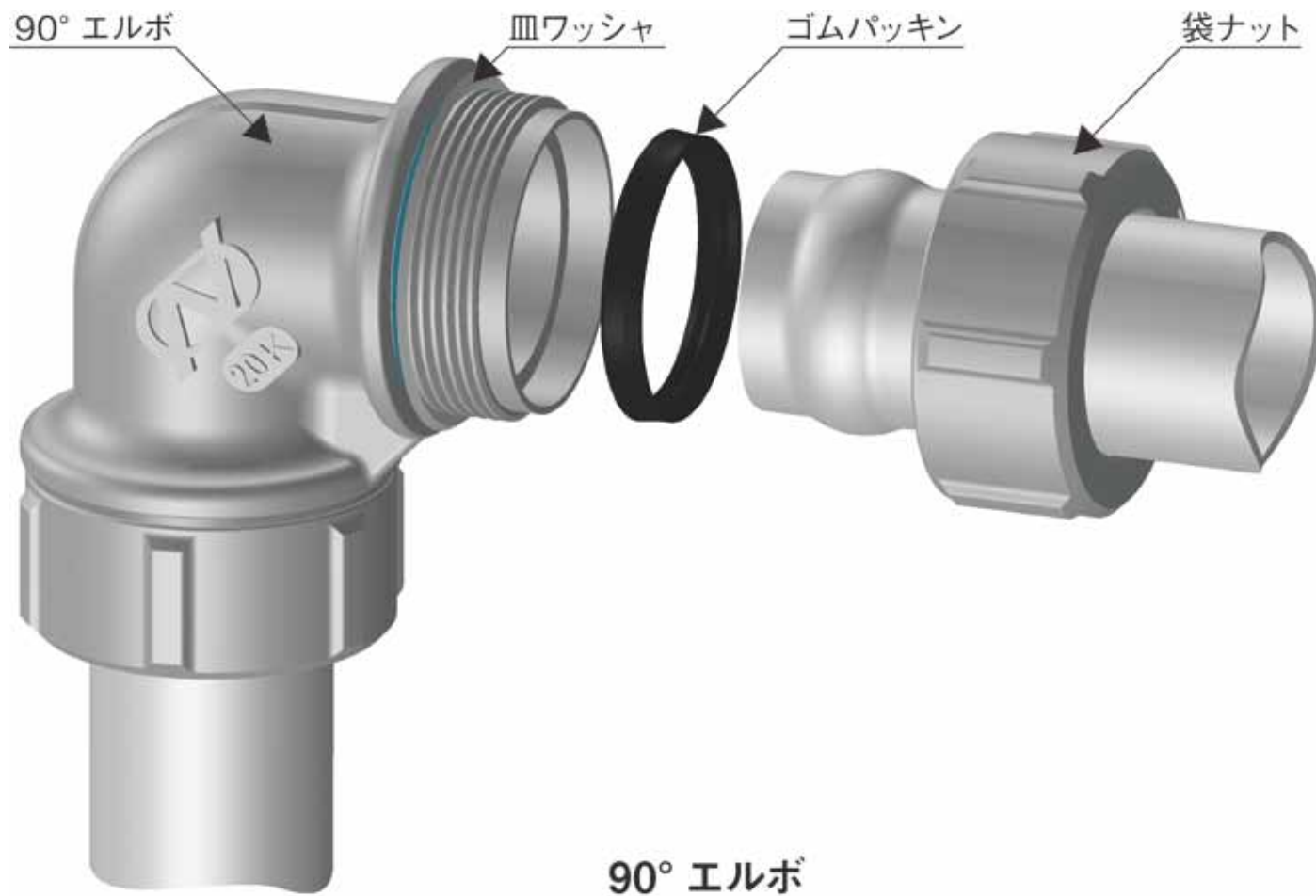
拡管式管継手(ナイスジョイント)13~60Su
