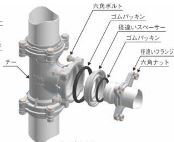
径違いチー
