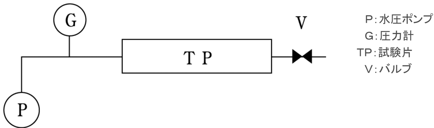
試験概要図
