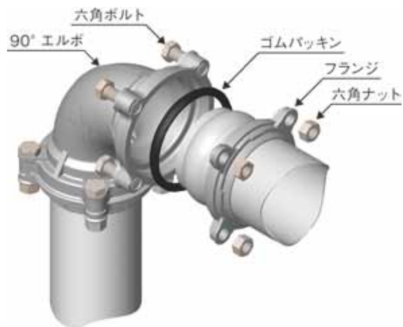
90° エルボ
