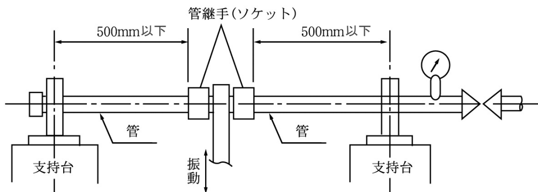
振動試験概要図
