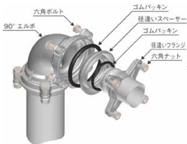
径違いエルボ
