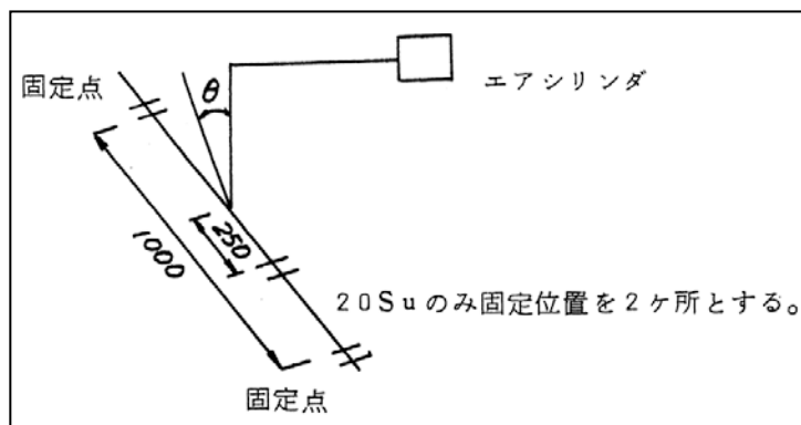
試験概要図
