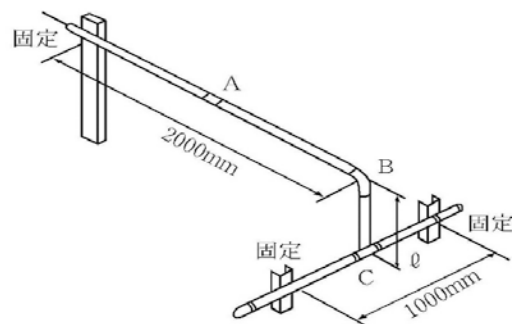
冷温水サイクル試験概要図
