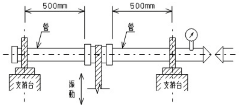
図1 耐震試験装置
