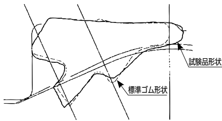
1年2か月経過品 (50Su 断面形状)
