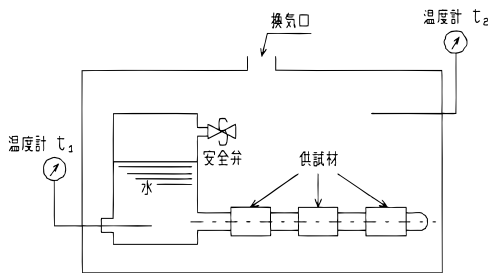
試験配管図
