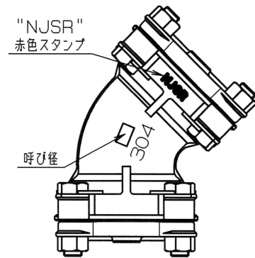
△ 外観図 (裏)
