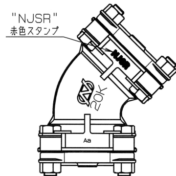
△ 外観図 (表)
