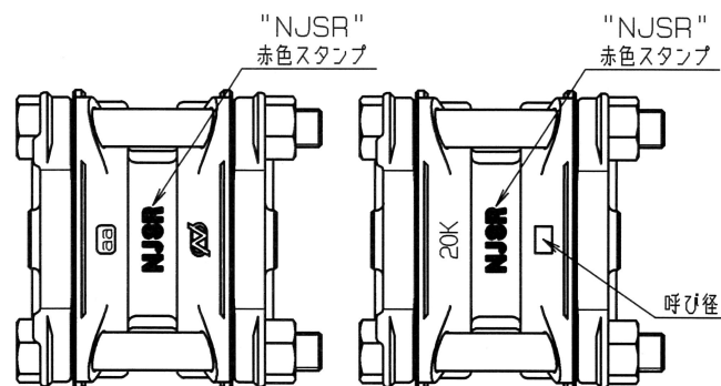
△外觀圖 (表)
