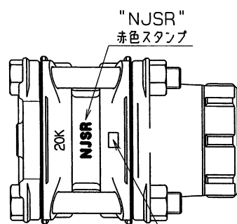
△ 外観図 (表)
