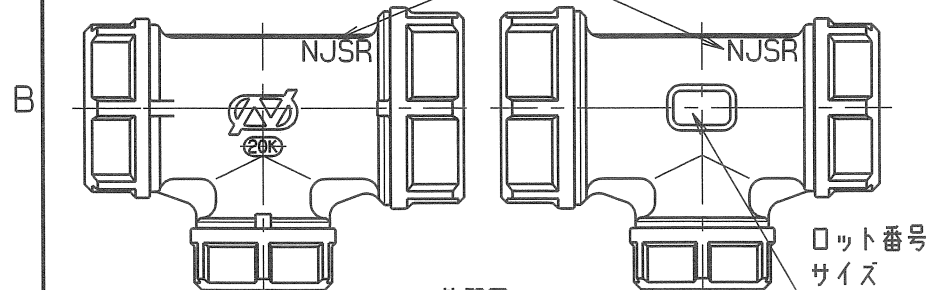
外観図
