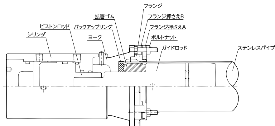
図8. 拡管機構
