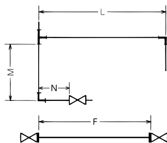
図10. 切断寸法表の使用例
