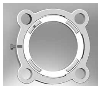
貫通フランジAをBに組み込む。
