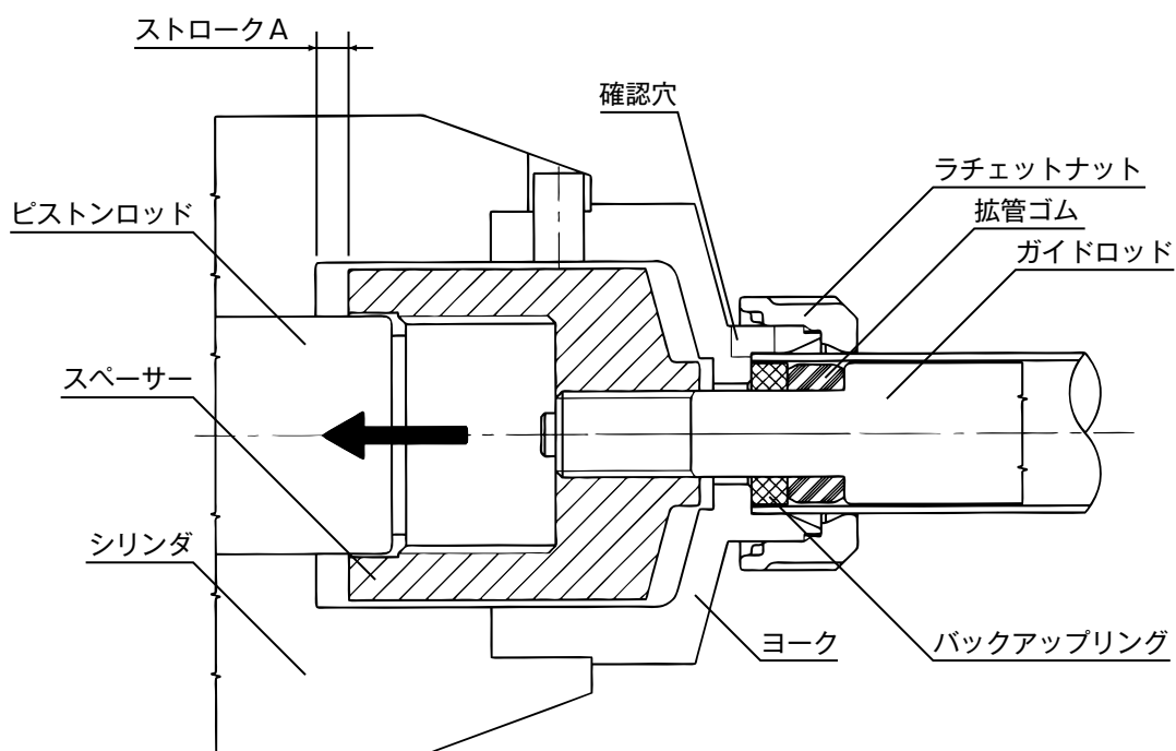
図2. 拡管機構
