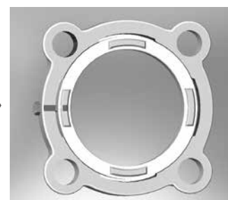
貫通フランジAとBの合印を合わせる。六角ボルトをすき間がなくなるまでしっかりと締め込む。
