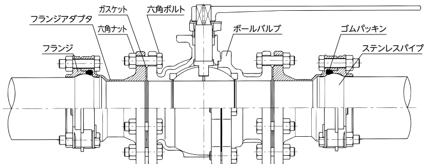
図7. JIS 10K フランジとの接続方法
