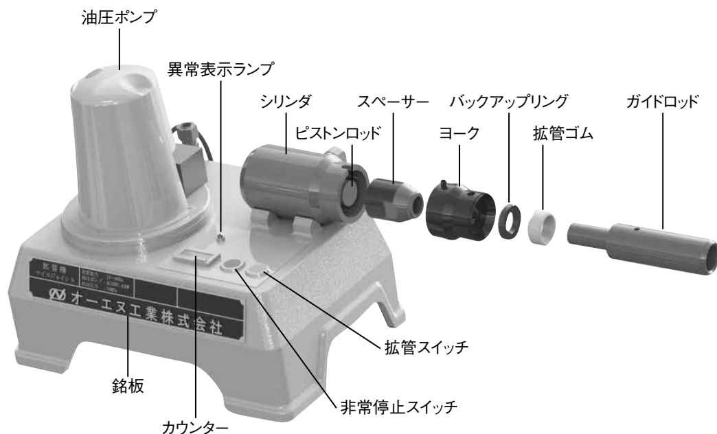
図3. NE500型拡管機組立図
