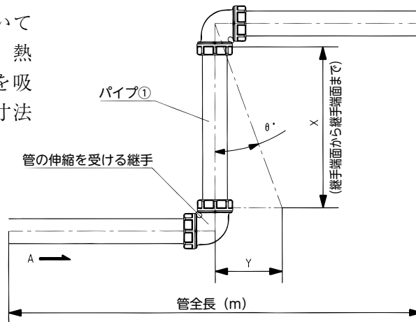
図13. 曲り配管 1ヶ
