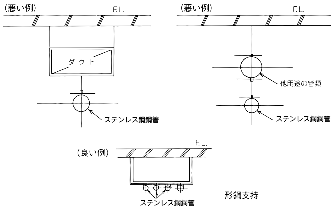
図11. 支持・固定要領 (参考資料：ステンレス協会編、建築用ステンレスマニュアルより)
