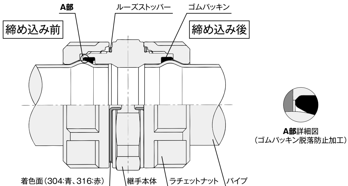
図1. 拡管式管継手(ナイスジョイントNJ-X) 呼び径: 13~60Suの構造
