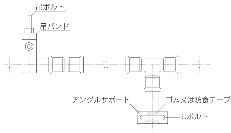
図2. 配管支持要領
