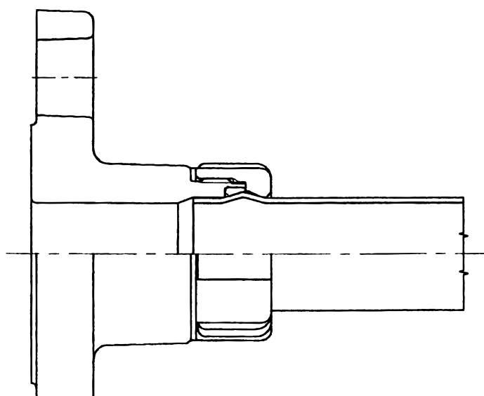
図2. 組立完成図
