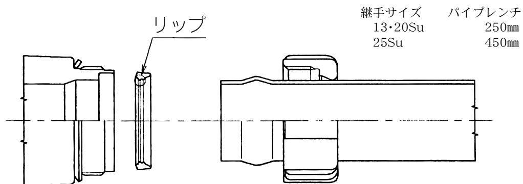
図1. 取り付け行程図
